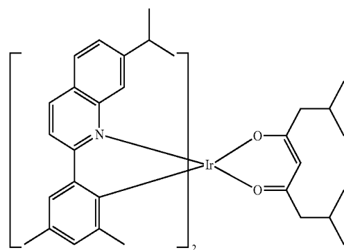
Compound E36
