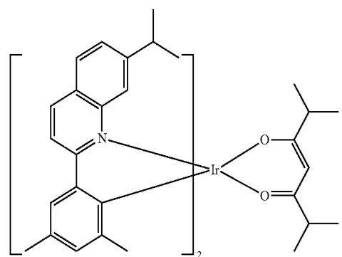
Compound E36
