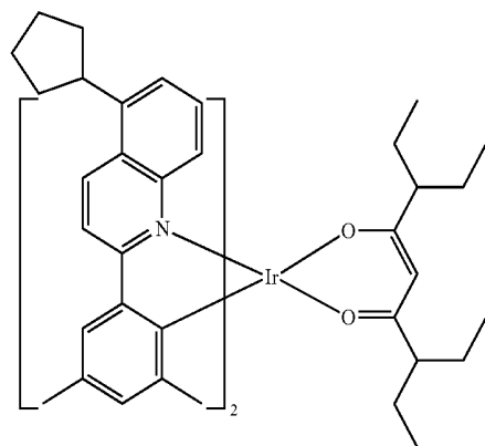
Compound E19
