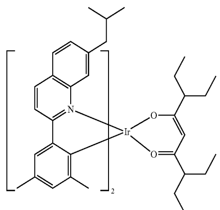
Compound E10
