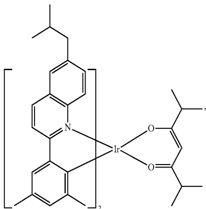
Compound E15
