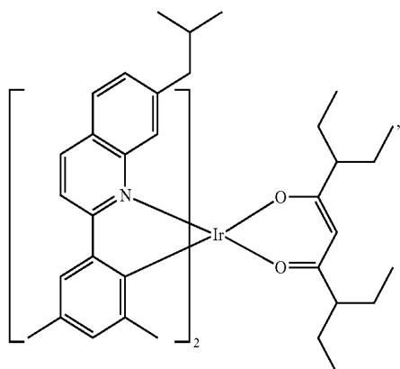
Compound E11
