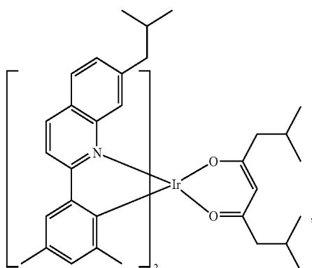
Compound E12
