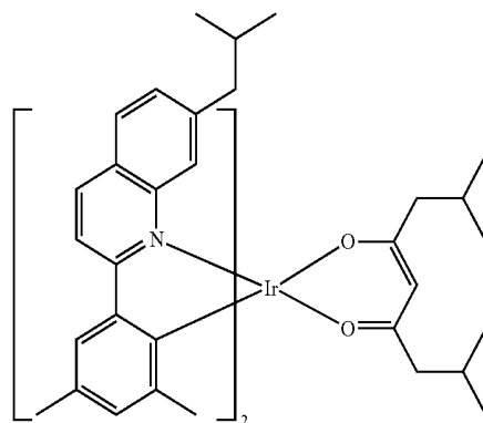
Compound E12
