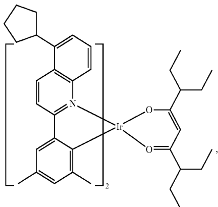
Compound E19
