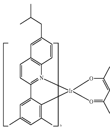
Compound E10
